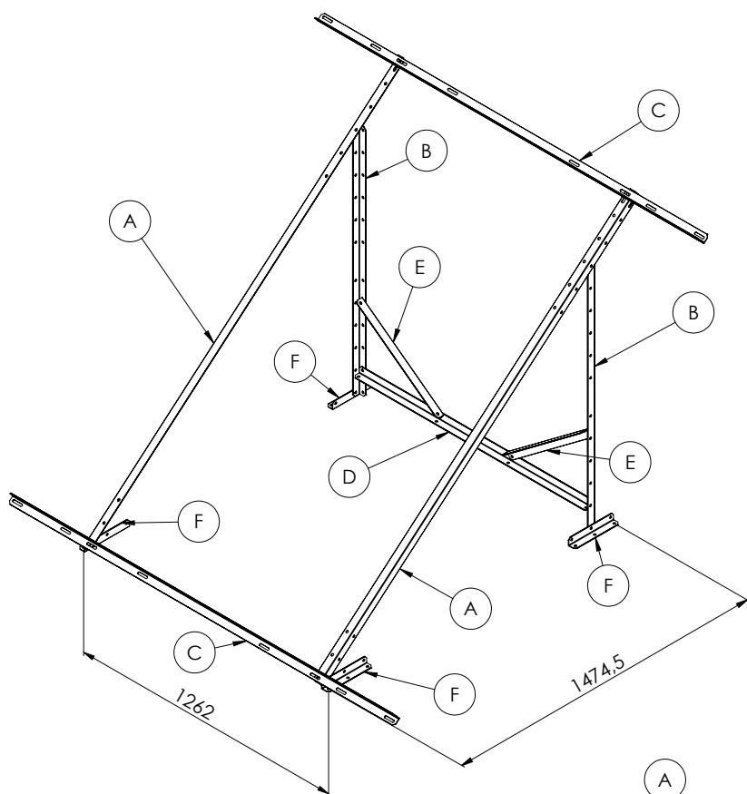
Cubierta plana
