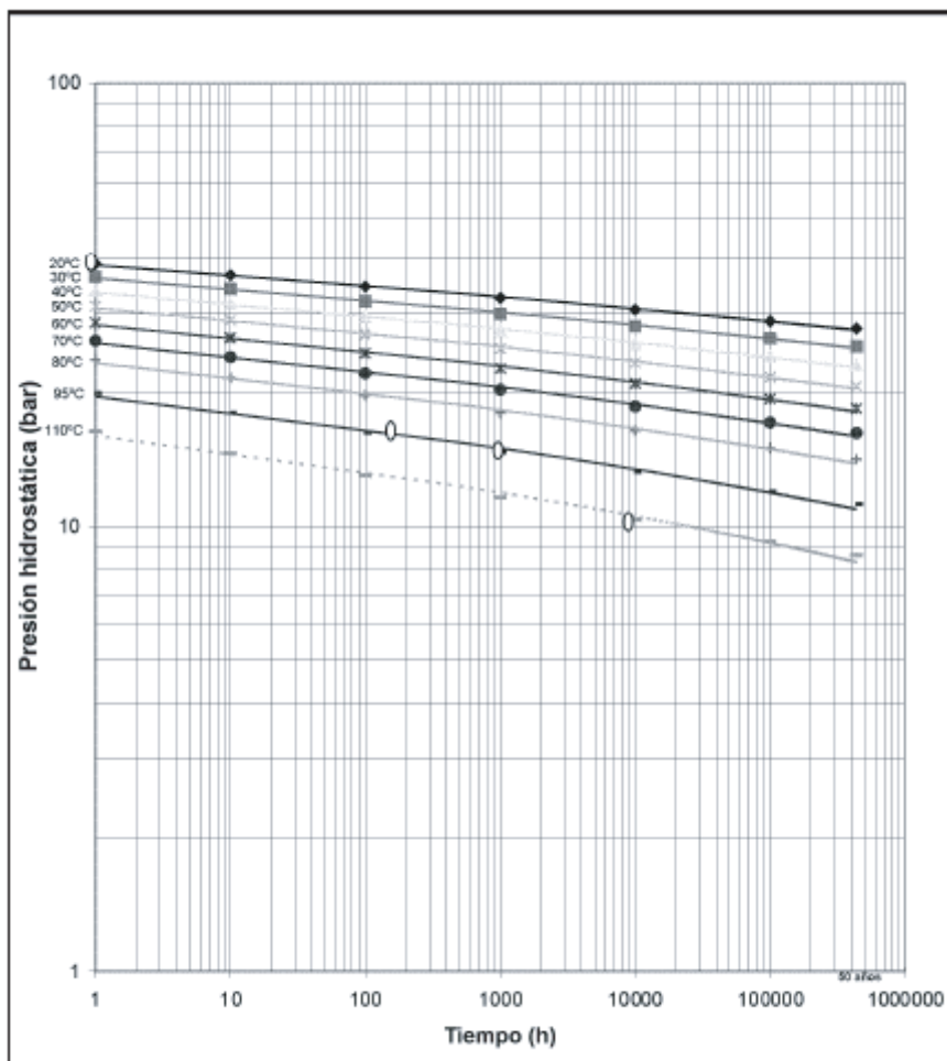
Curvas de referencia mínimas de los tubos multicapa Polímero/AL/PEX
