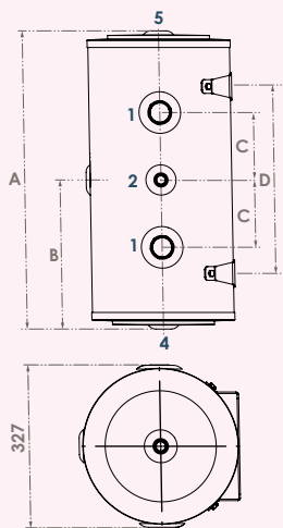
INA30-50: Instalación mural vertical y horizontal. Apto para exteriores
