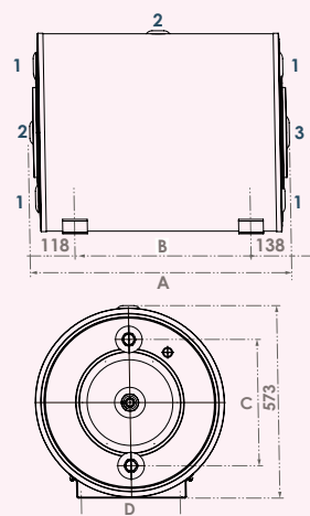
INA50H-100H: Instalación mural vertical y horizontal y suelo horizontal. Apto para exteriores.
